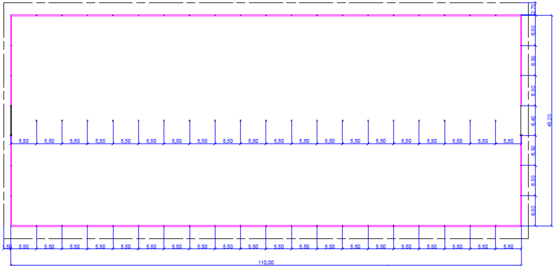
PLANTA BAIXA
