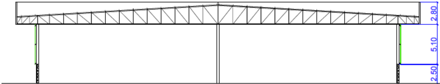
CORTE
